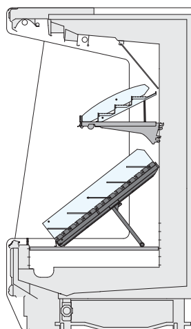
Divisore verticale per griglia areata H 125 mm Materiale: PMMA spessore 5 mm
