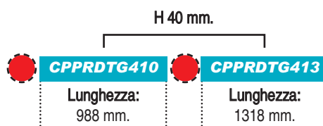
Profilo porta prezzo Tegometall P50 doppia altezza.
