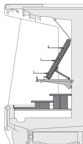
Divisore verticale per griglia areata H 175 mm Materiale: PMMA spessore 5 mm
